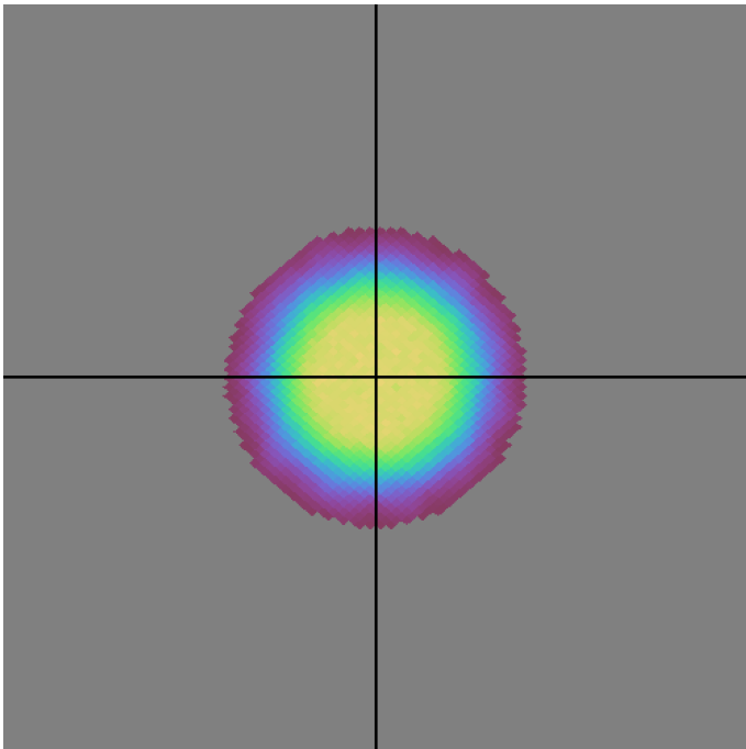
roman_v3.3_10yrs r band: DD:COSMOS NVisits
