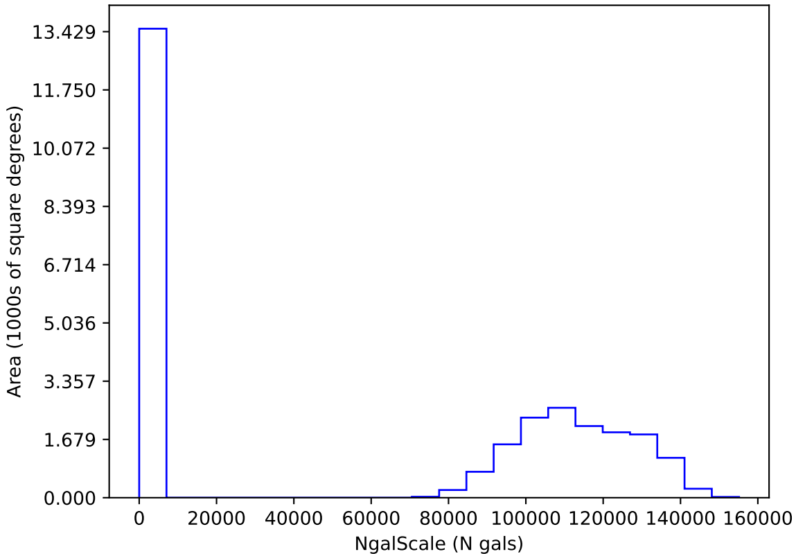
roll_uniform_eh_acc0.8_mjdp0_v3.4_10yrs i: NgalScale
