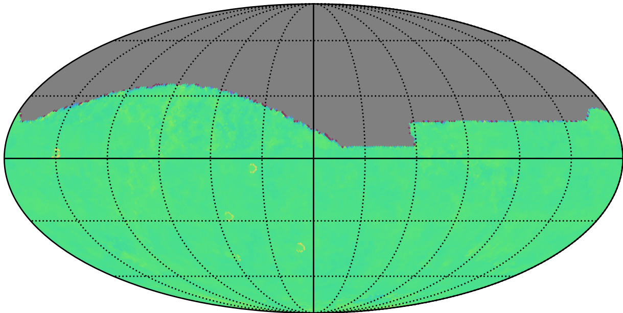
roll_uniform_eh_acc0.8_mjdp0_v3.4_10yrs z: Kuiper rotTelPos
