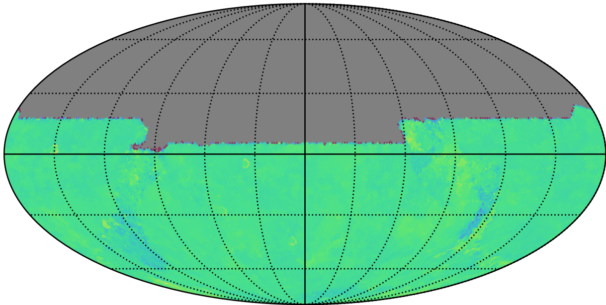
roll_uniform_eh_acc0.8_mjdp0_v3.4_10yrs u: Kuiper rotTelPos
