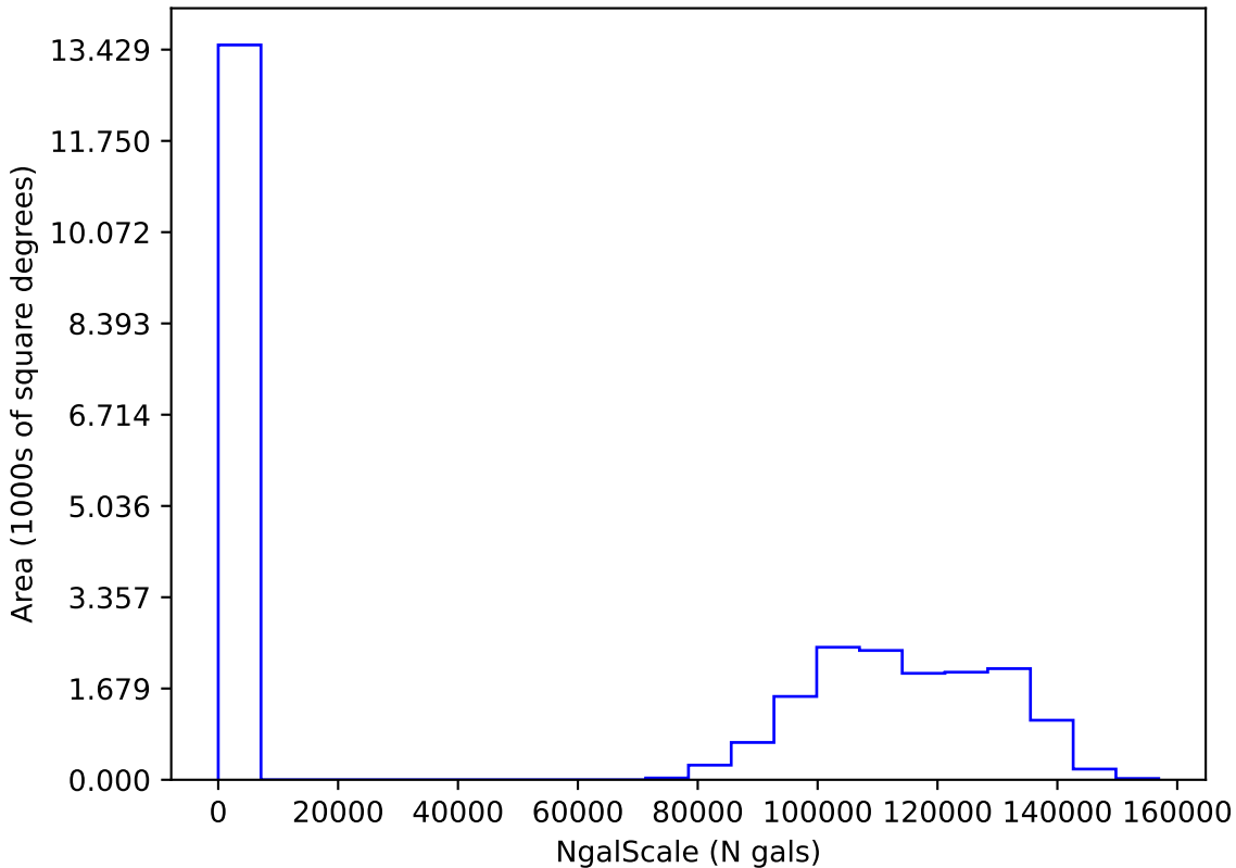
roll_uniform_eh_acc0.2_mjdp0_v3.4_10yrs i: NgalScale
