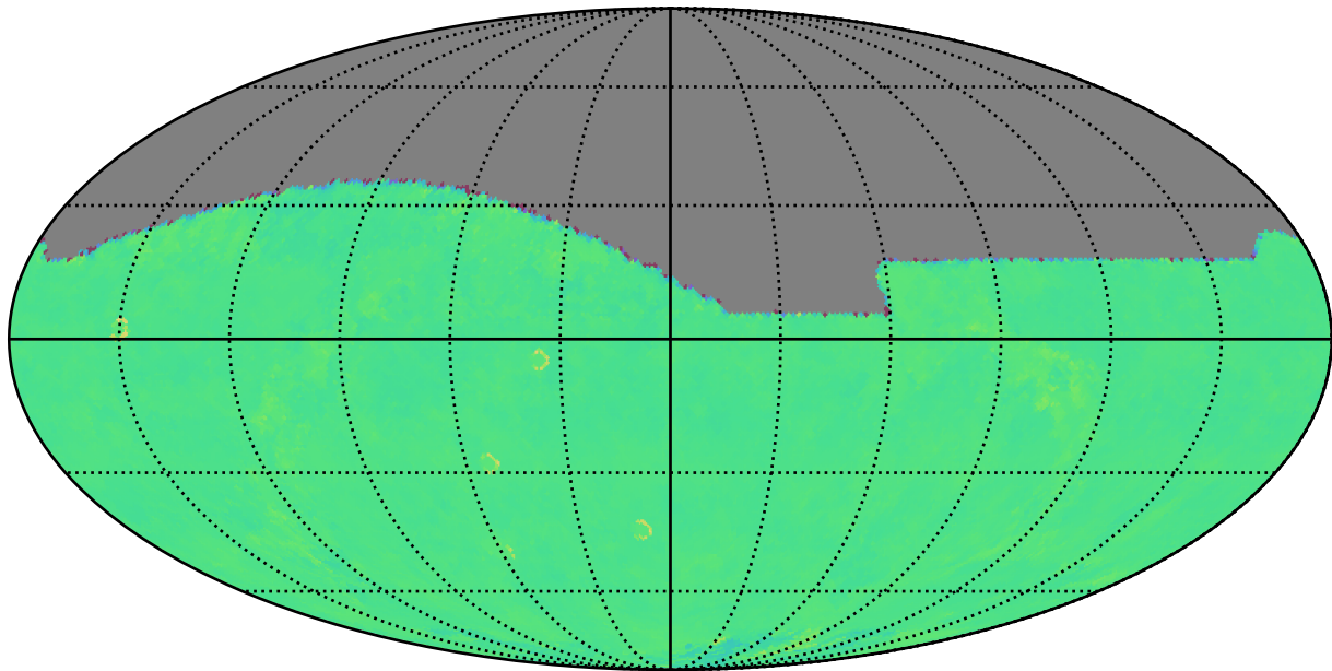
roll_uniform_early_half_mjdp67_v3.4_10yrs z: Kuiper rotTelPos
