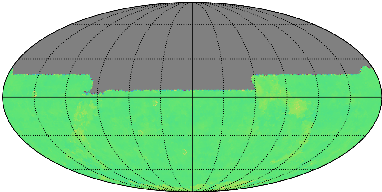
roll_uniform_early_half_mjdp67_v3.4_10yrs y: Kuiper rotTelPos
