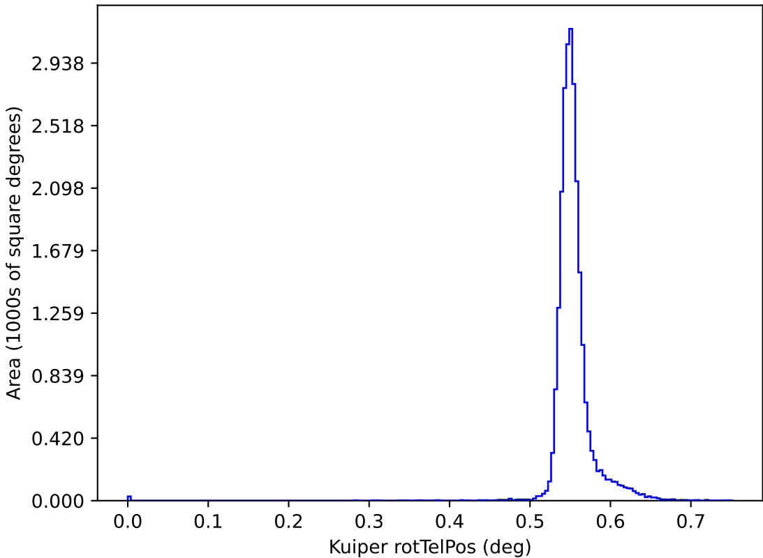
roll_uniform_early_half_mjdp67_v3.4_10yrs y: Kuiper rotTelPos
