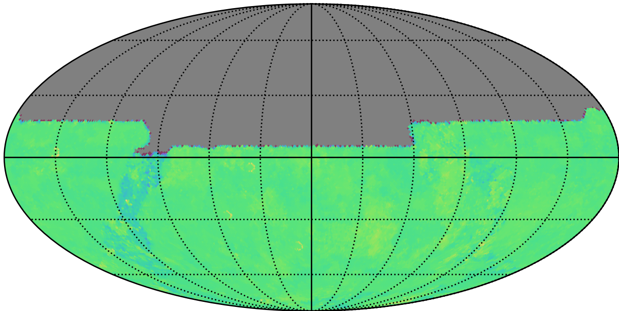
roll_uniform_early_half_mjdp67_v3.4_10yrs u: Kuiper rotTelPos
