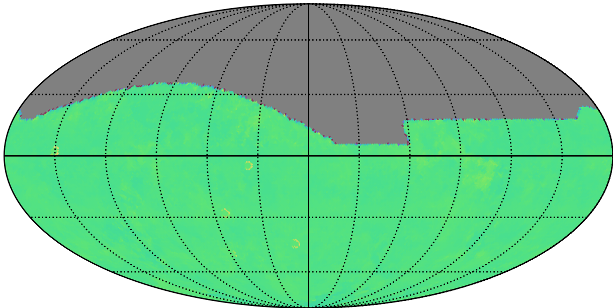
roll_uniform_early_half_mjdp67_v3.4_10yrs i: Kuiper rotTelPos
