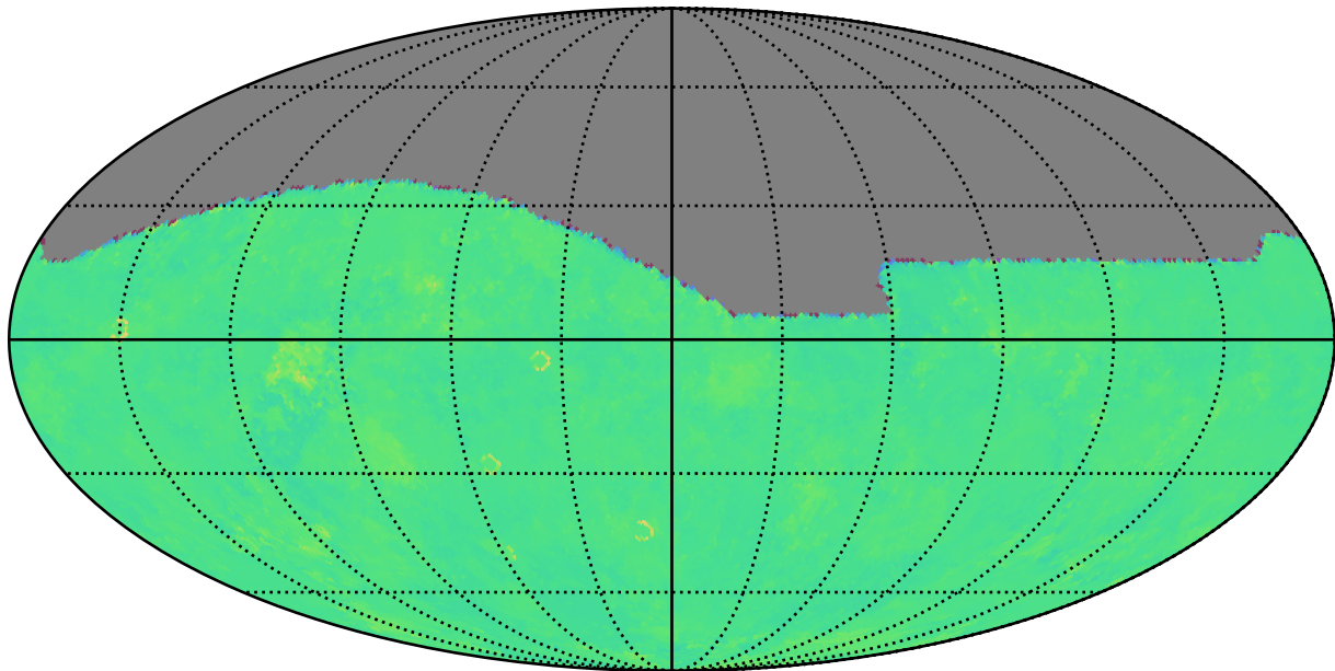
roll_uniform_early_half_mjdp67_v3.4_10yrs g: Kuiper rotTelPos
