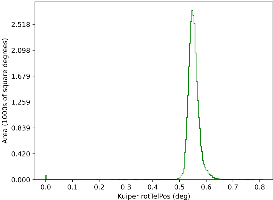
roll_uniform_early_half_mjdp67_v3.4_10yrs g: Kuiper rotTelPos
