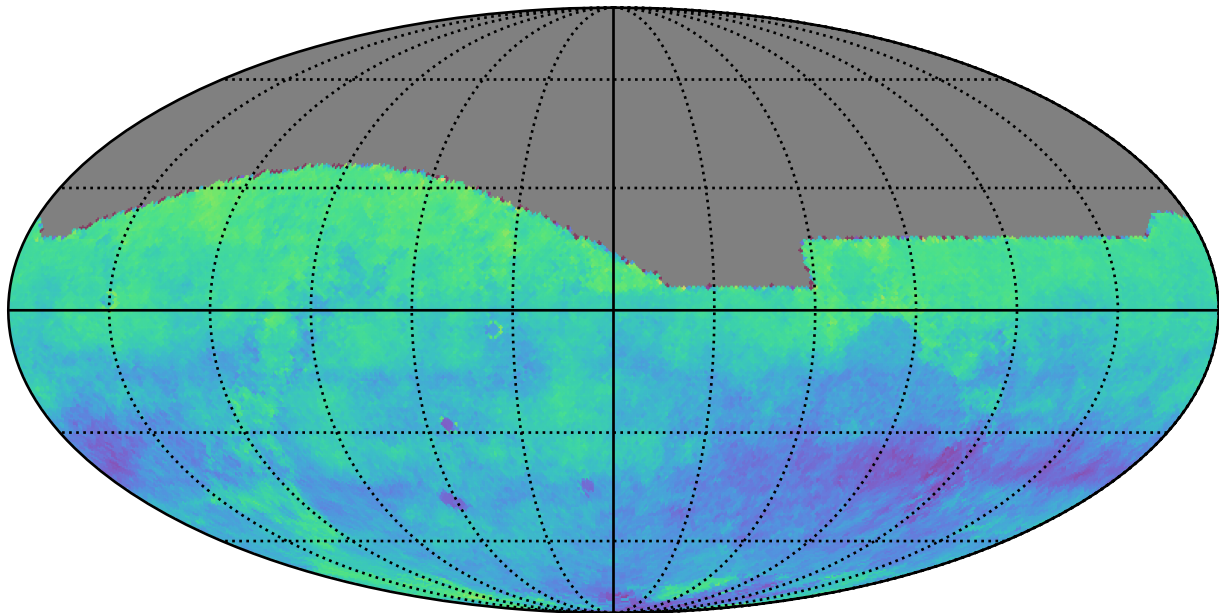
roll_uniform_early_half_mjdp67_v3.4_10yrs i: Kuiper rotSkyPos
