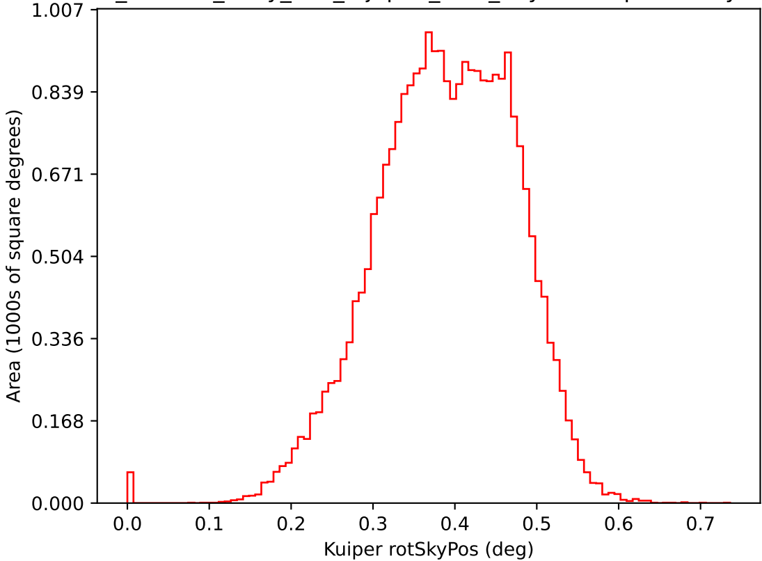
roll_uniform_early_half_mjdp67_v3.4_10yrs i: Kuiper rotSkyPos
