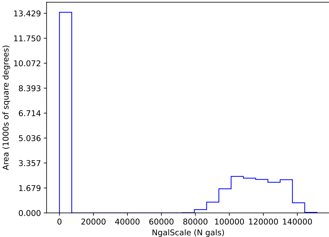
roll_uniform_early_half_mjdp253_v3.4_10yrs i: NgalScale
