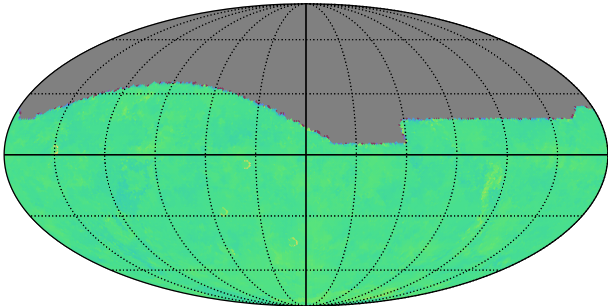
roll_uniform_early_half_mjdp253_v3.4_10yrs g: Kuiper rotTelPos
