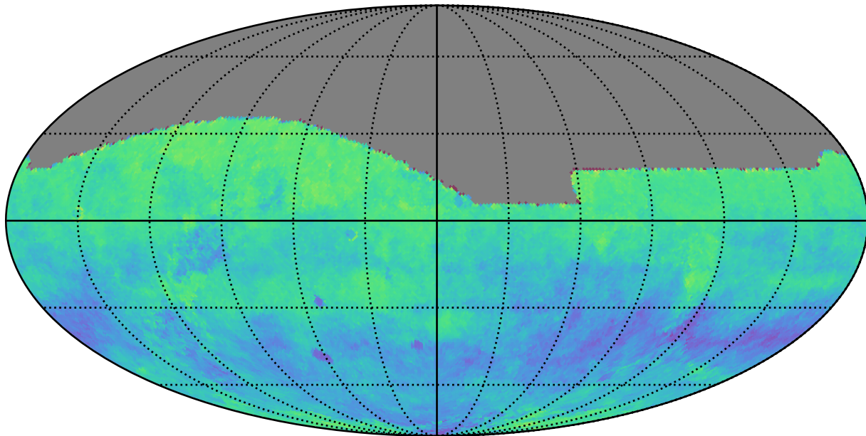
roll_uniform_early_half_mjdp253_v3.4_10yrs i: Kuiper rotSkyPos
