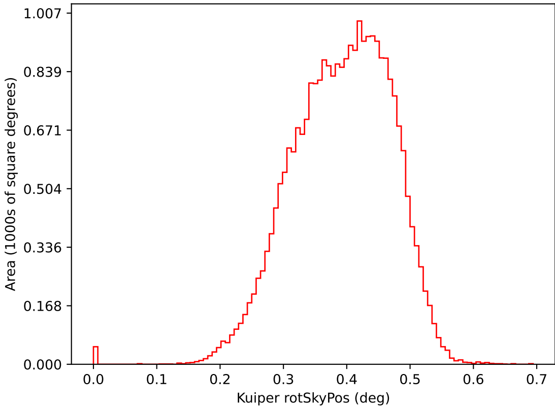
roll_uniform_early_half_mjdp253_v3.4_10yrs i: Kuiper rotSkyPos
