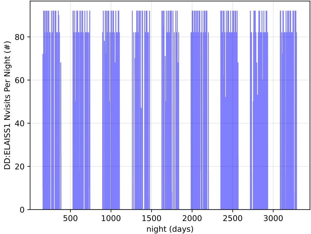
roll_uniform_early_half_mjdp253_v3.4_10yrs all bands: DD:ELAISS1 Nvisits Per Night
