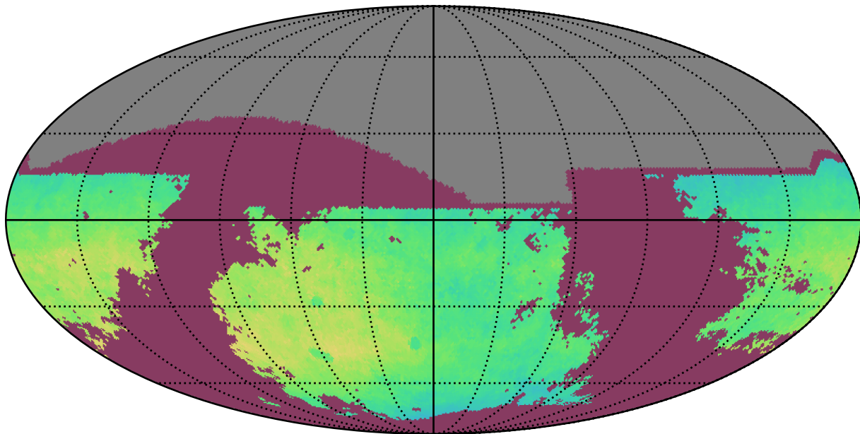
roll_uniform_early_half_mjdp180_v3.4_10yrs i: NgalScale
