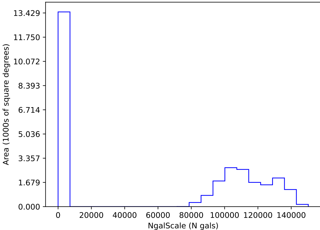
roll_uniform_early_half_mjdp180_v3.4_10yrs i: NgalScale
