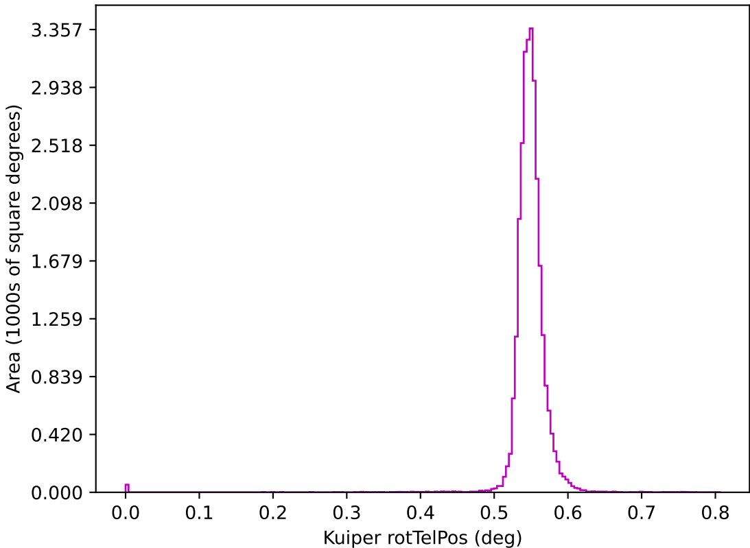
roll_uniform_early_half_mjdp180_v3.4_10yrs z: Kuiper rotTelPos
