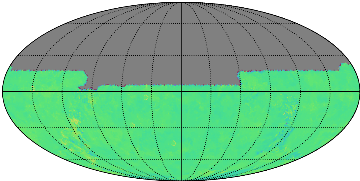
roll_uniform_early_half_mjdp180_v3.4_10yrs u: Kuiper rotTelPos
