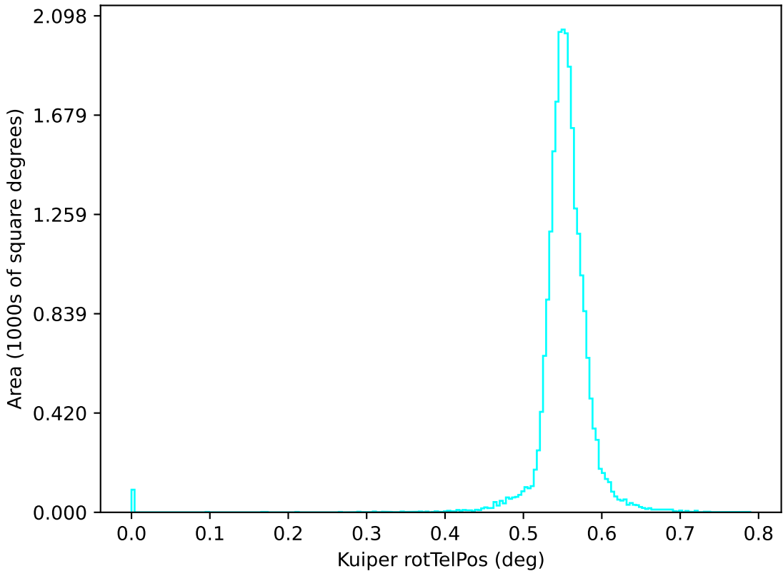
roll_uniform_early_half_mjdp180_v3.4_10yrs u: Kuiper rotTelPos
