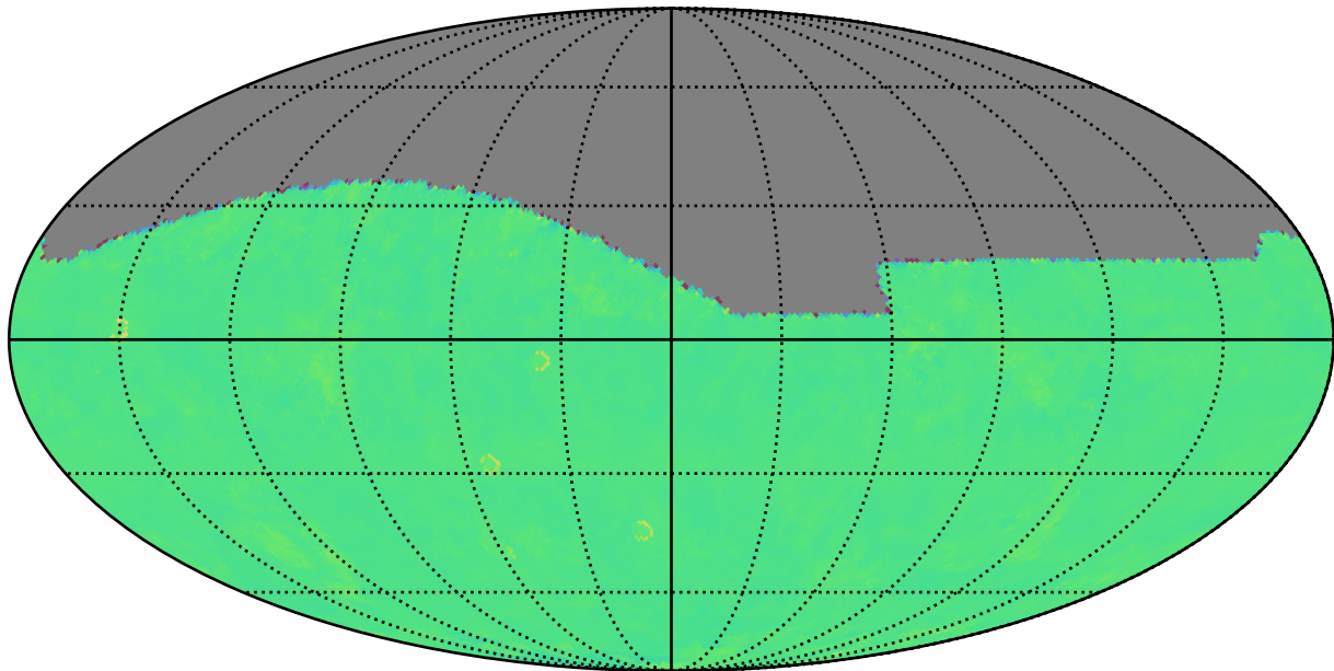
roll_uniform_early_half_mjdp180_v3.4_10yrs i: Kuiper rotTelPos
