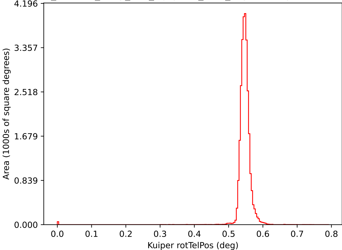
roll_uniform_early_half_mjdp180_v3.4_10yrs i: Kuiper rotTelPos
