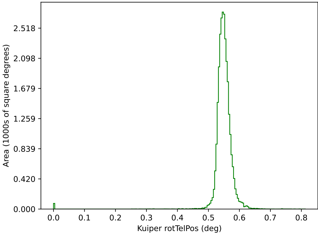
roll_uniform_early_half_mjdp180_v3.4_10yrs g: Kuiper rotTelPos
