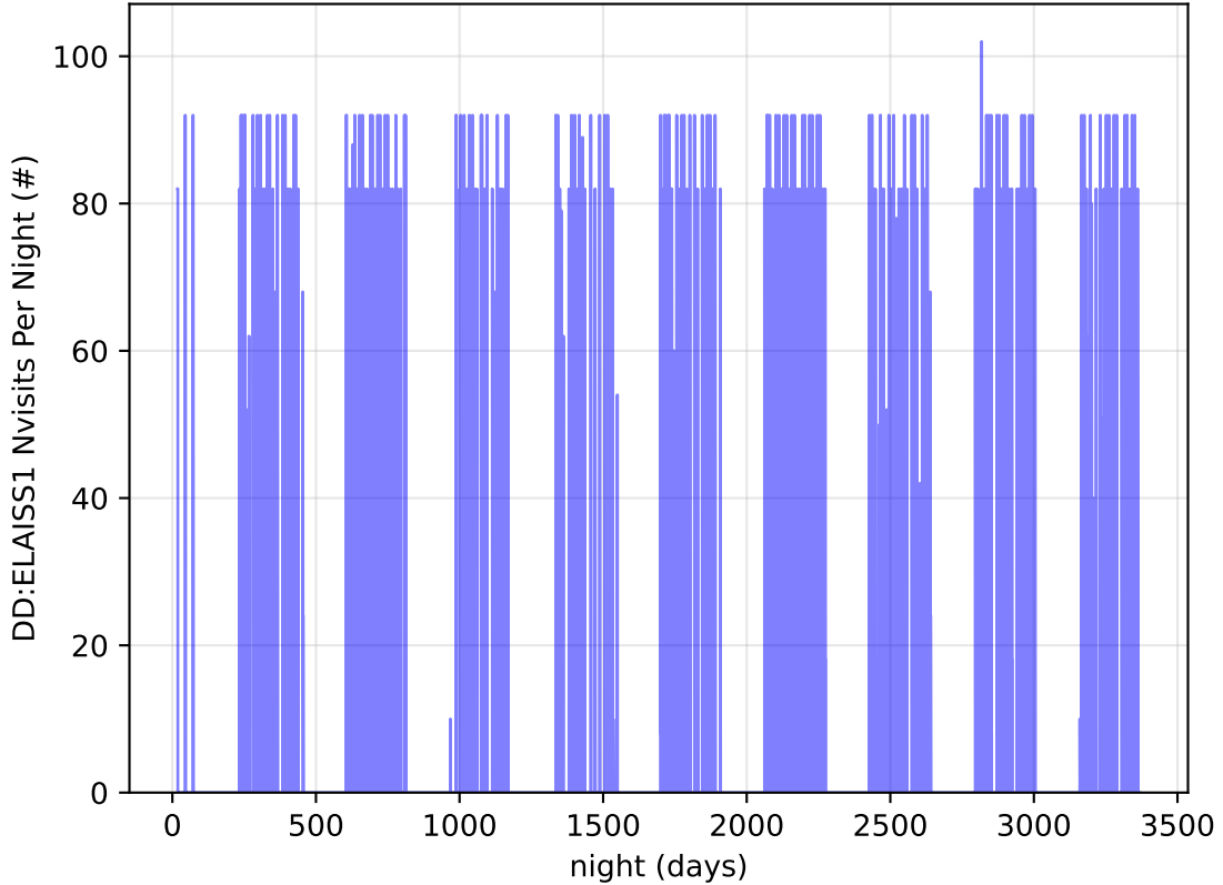
roll_uniform_early_half_mjdp180_v3.4_10yrs all bands: DD:ELAISS1 Nvisits Per Night
