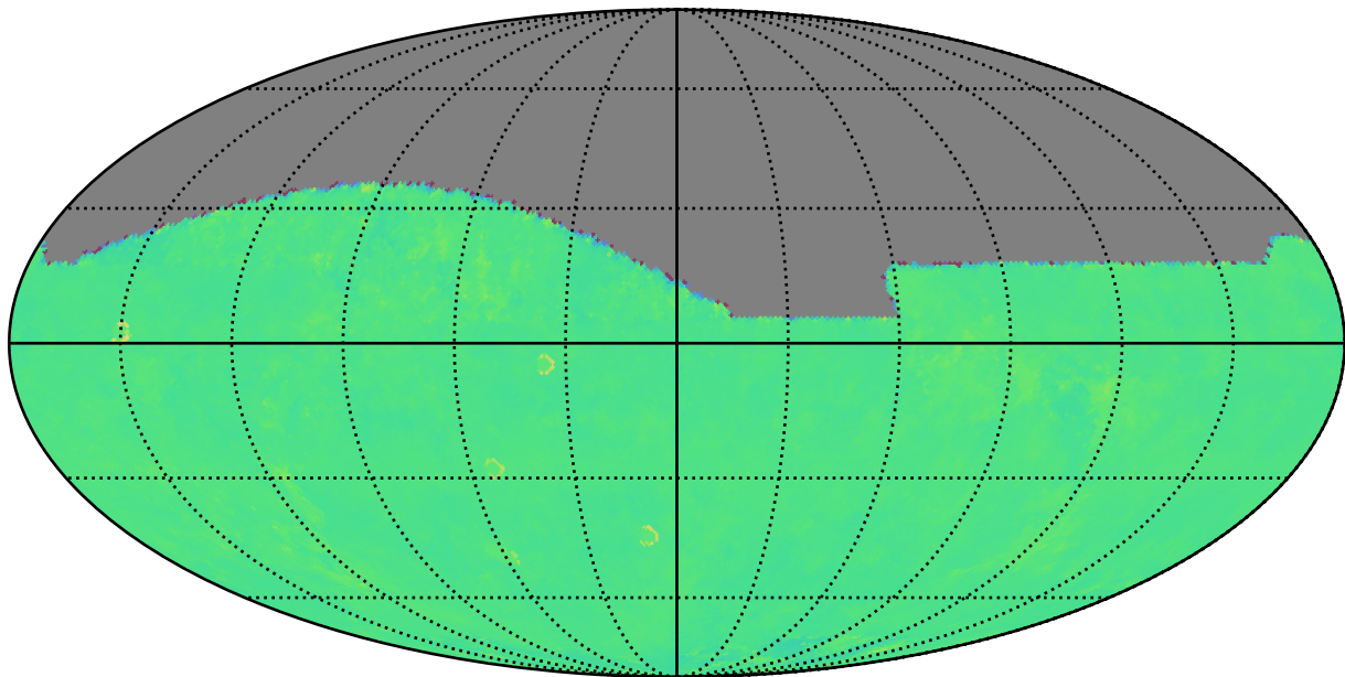
roll_uniform_early_half_mjdp0_v3.4_10yrs z: Kuiper rotTelPos
