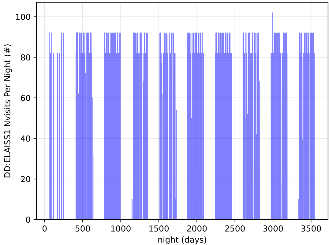
roll_uniform_early_half_mjdp0_v3.4_10yrs all bands: DD:ELAISS1 Nvisits Per Night
