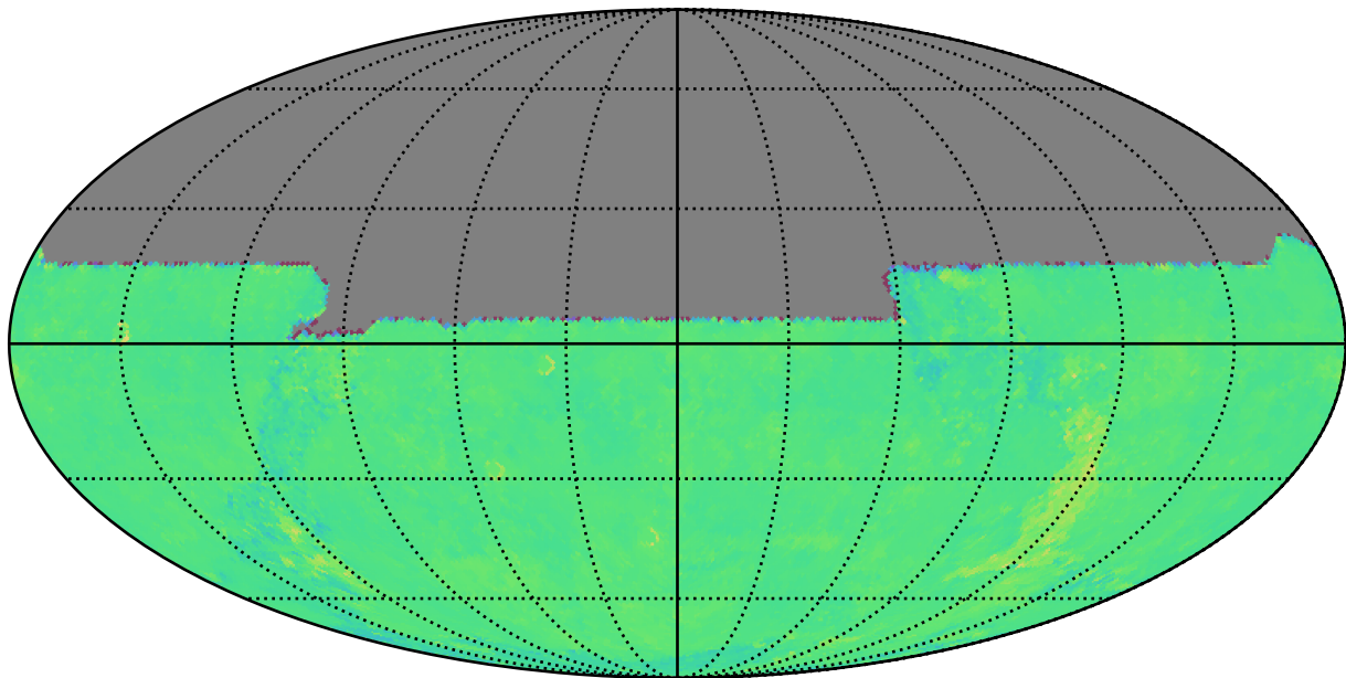
roll_pause_mjdp60_v3.4_10yrs u: Kuiper rotTelPos
