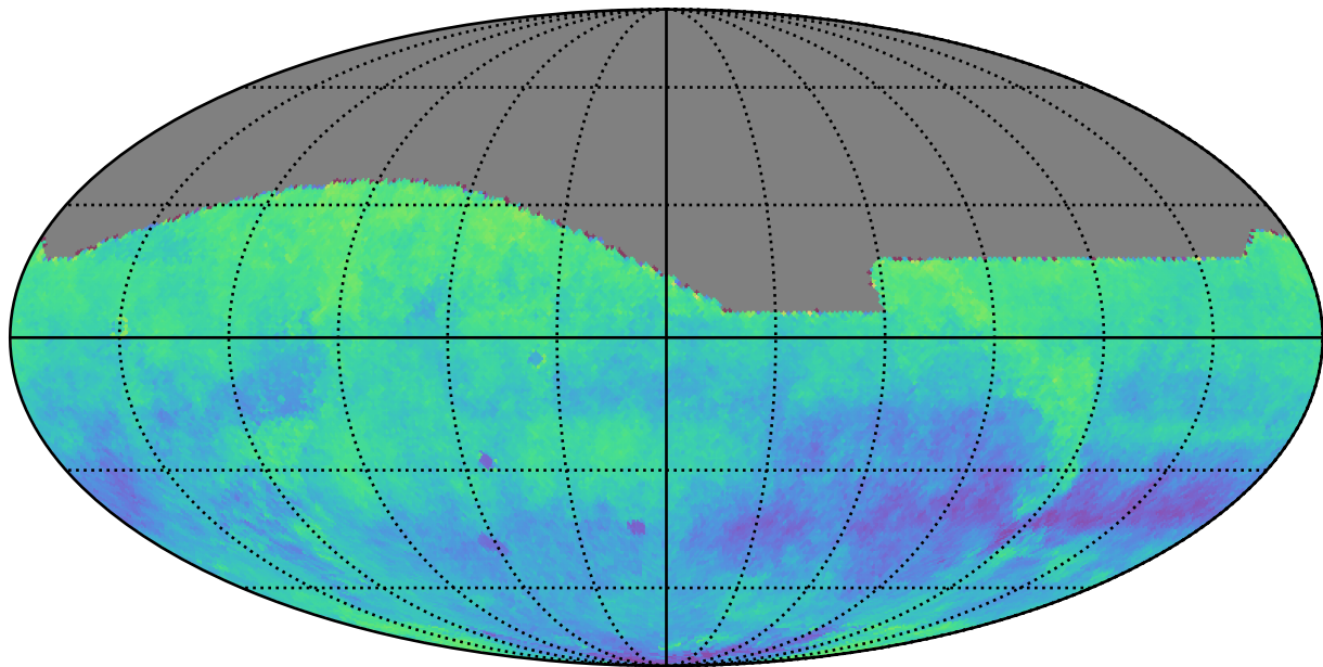
roll_pause_mjdp60_v3.4_10yrs i: Kuiper rotSkyPos
