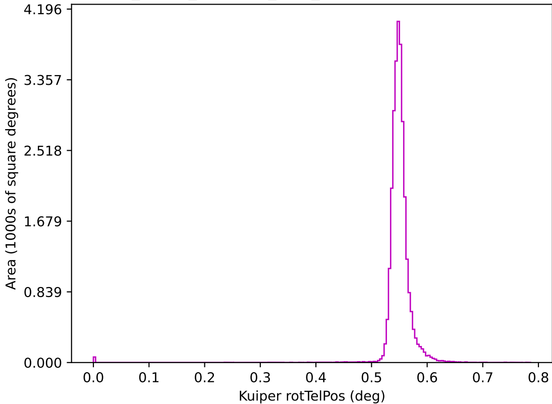
roll_pause_mjdp365_v3.4_10yrs z: Kuiper rotTelPos
