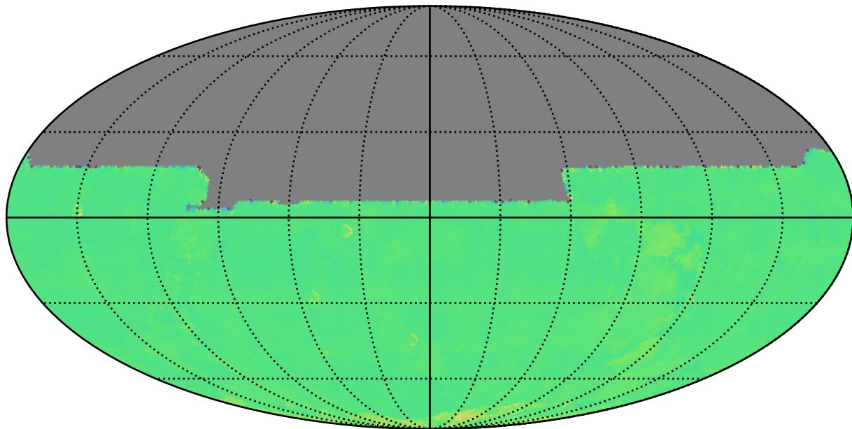
roll_pause_mjdp365_v3.4_10yrs y: Kuiper rotTelPos
