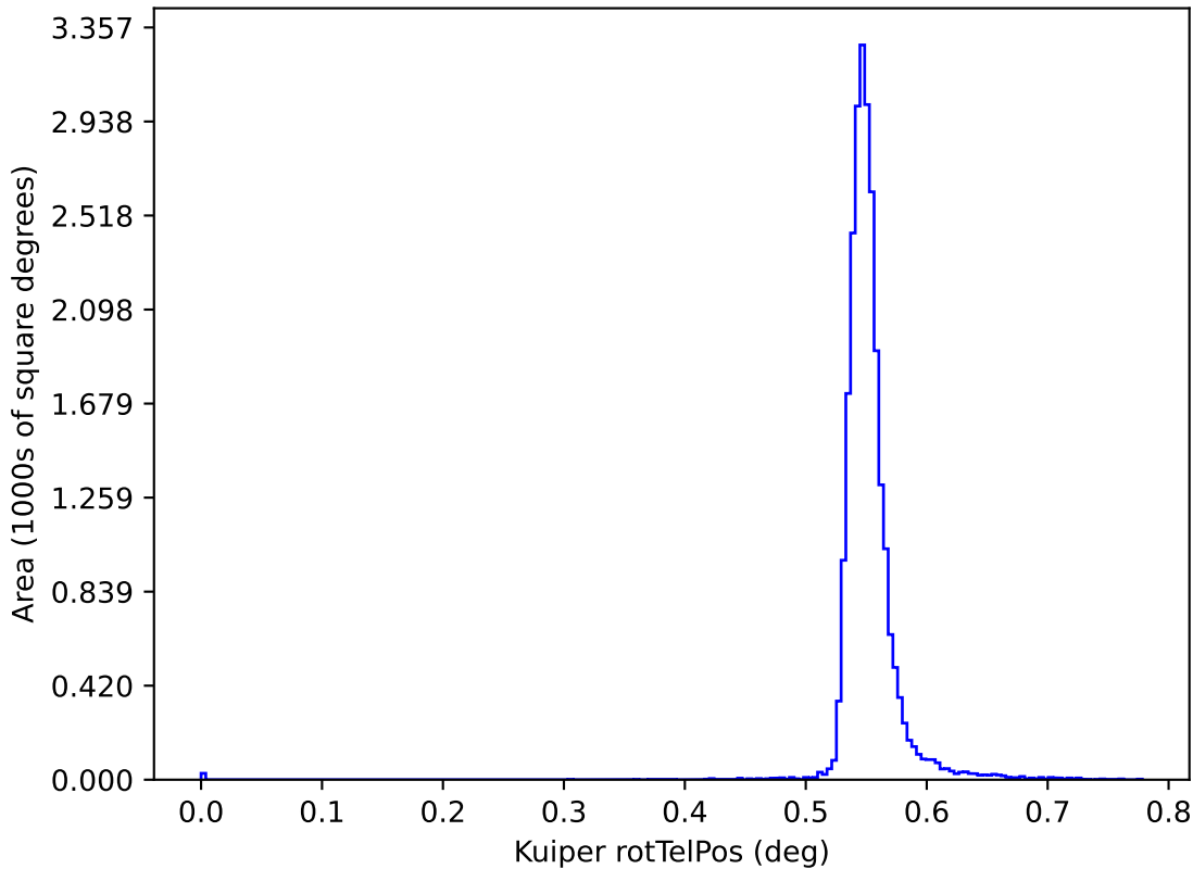
roll_pause_mjdp365_v3.4_10yrs y: Kuiper rotTelPos
