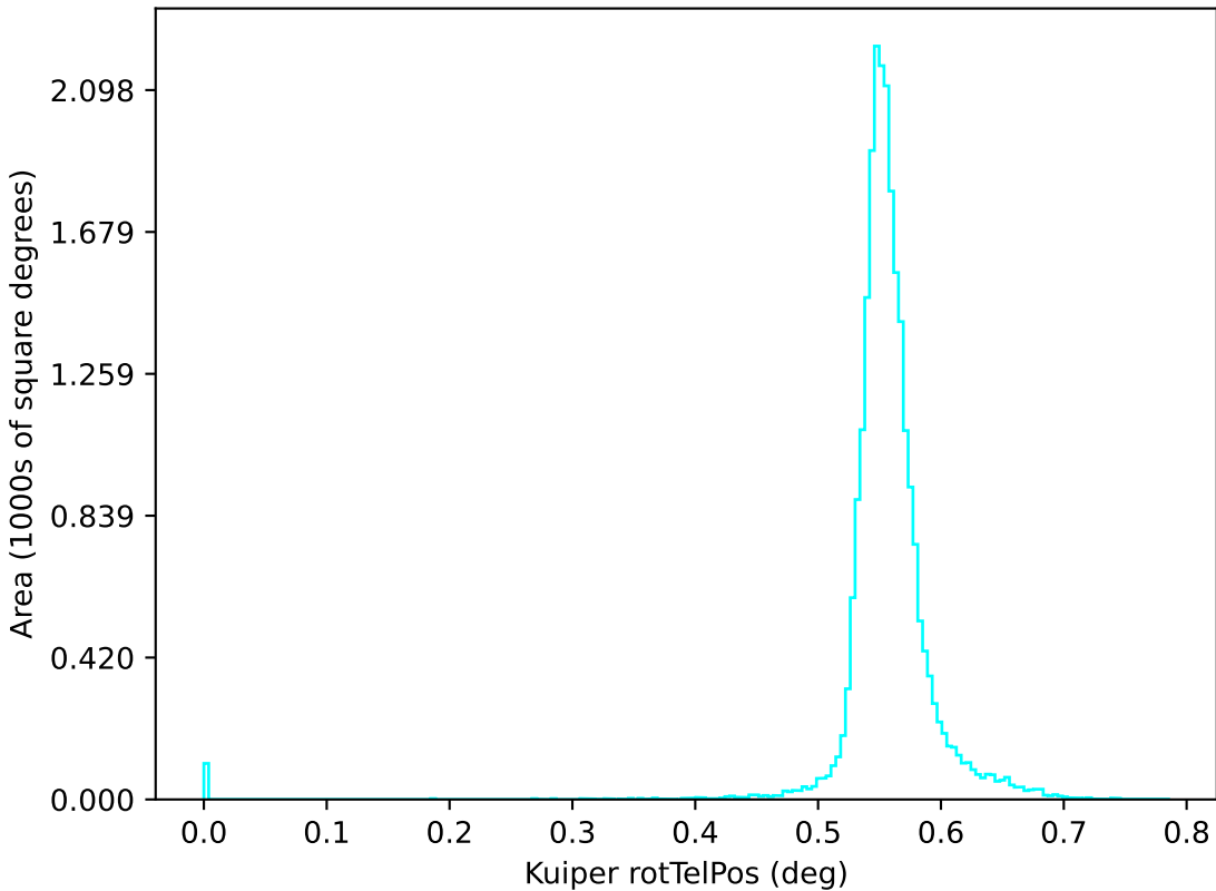
roll_pause_mjdp365_v3.4_10yrs u: Kuiper rotTelPos
