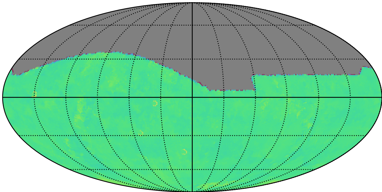
roll_pause_mjdp365_v3.4_10yrs g: Kuiper rotTelPos
