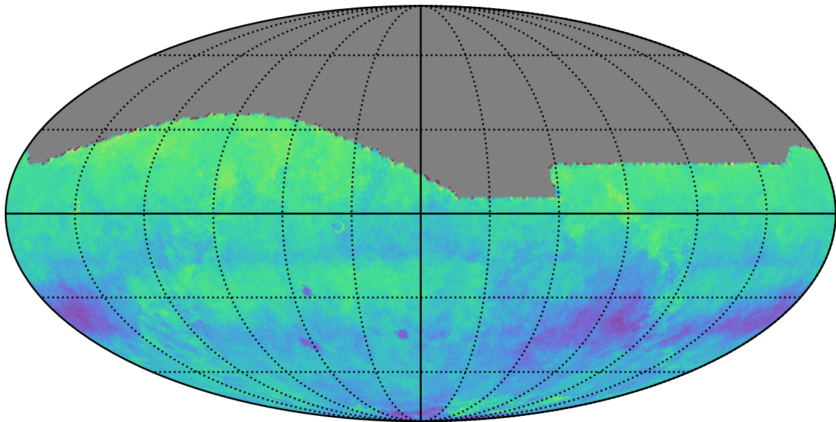
roll_pause_mjdp365_v3.4_10yrs i: Kuiper rotSkyPos
