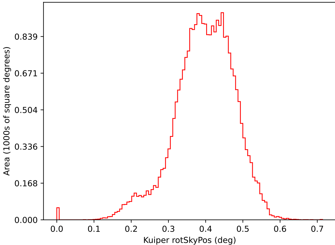
roll_pause_mjdp365_v3.4_10yrs i: Kuiper rotSkyPos
