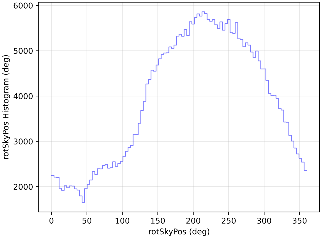
roll_pause_mjdp365_v3.4_10yrs WFD y band: rotSkyPos Histogram
