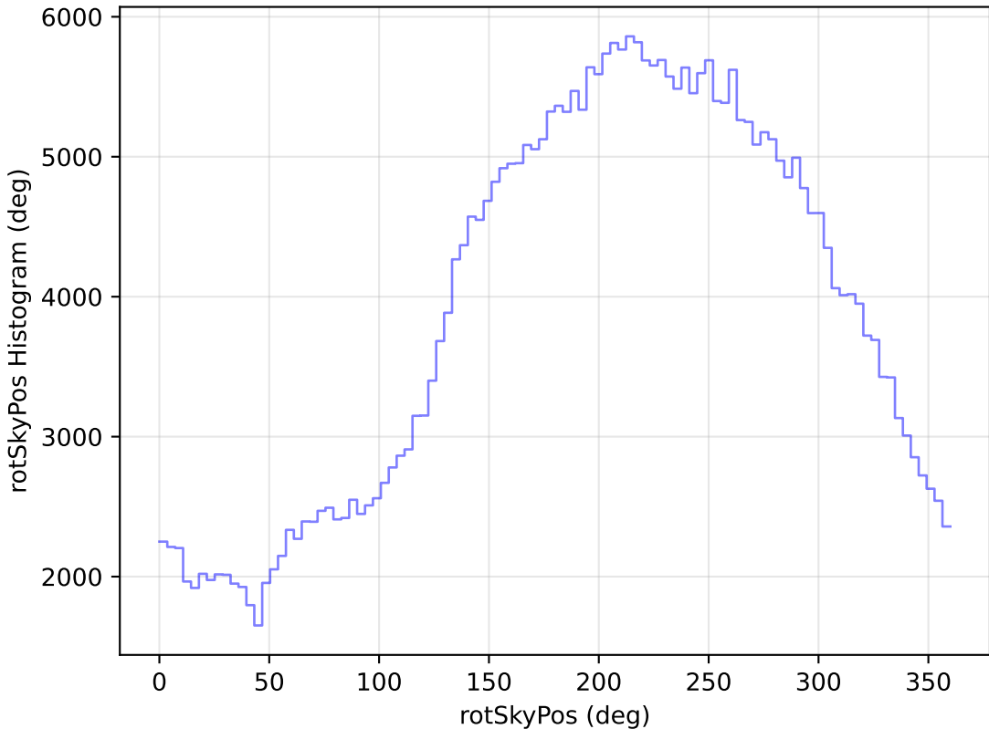
roll_pause_mjdp365_v3.4_10yrs All sky y band: rotSkyPos Histogram
