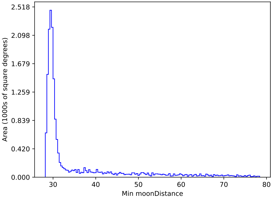
roll_pause_mjdp365_v3.4_10yrs WFD y band: Min moonDistance
