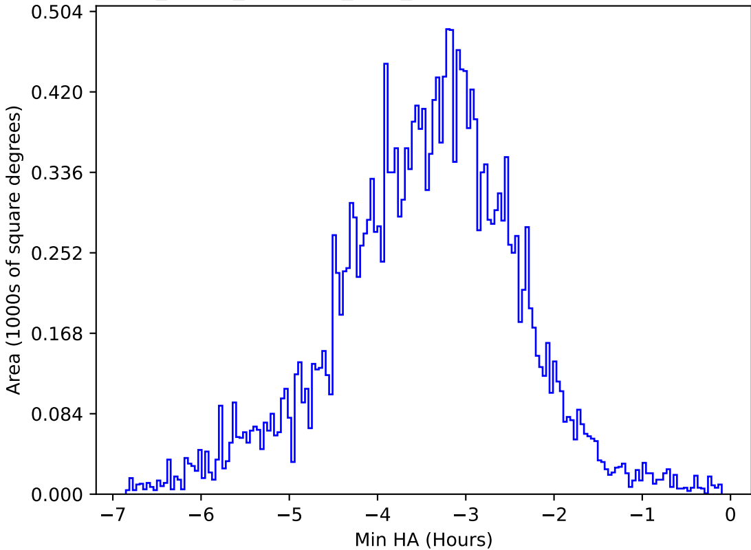
roll_pause_mjdp365_v3.4_10yrs All sky y band: Min HA
