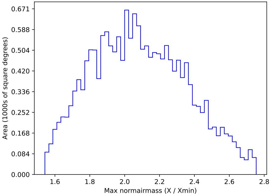
roll_pause_mjdp365_v3.4_10yrs WFD y band: Max normairmass
