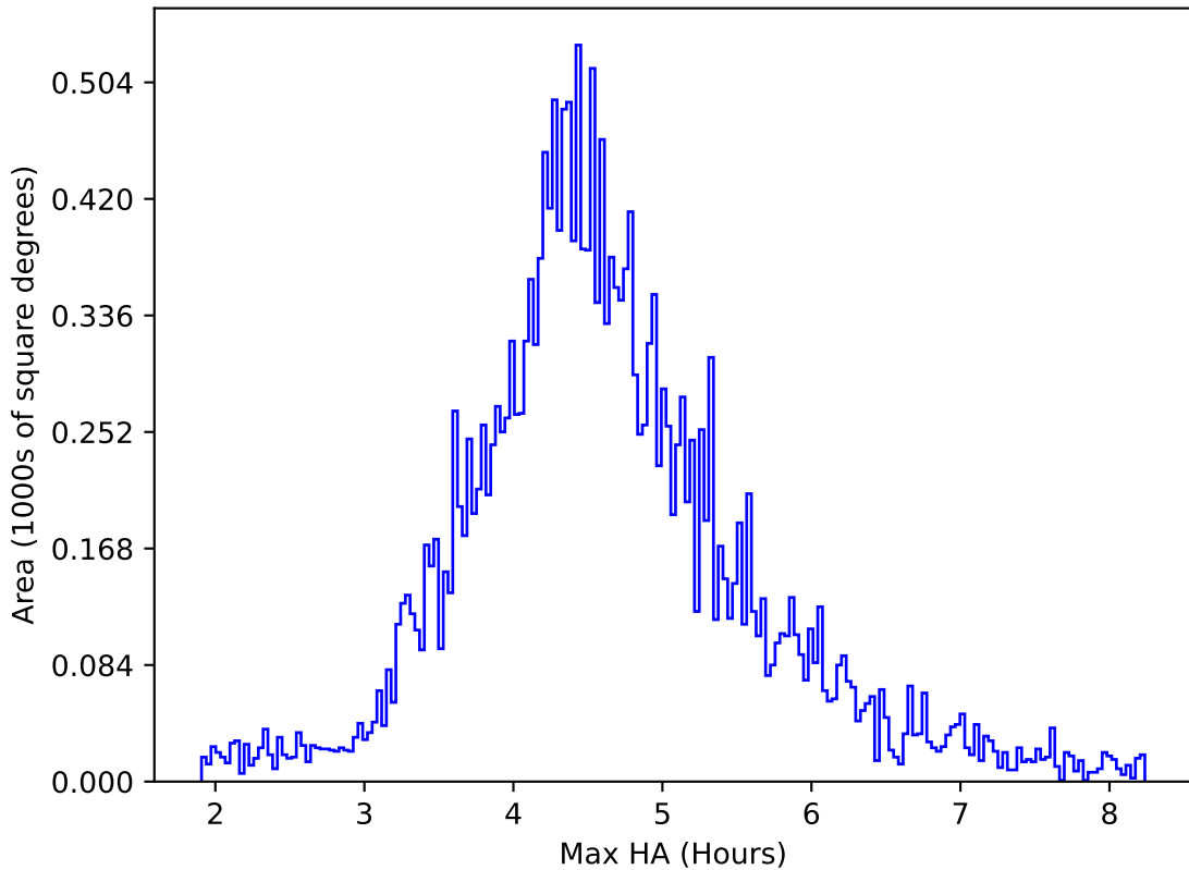
roll_pause_mjdp365_v3.4_10yrs All sky y band: Max HA
