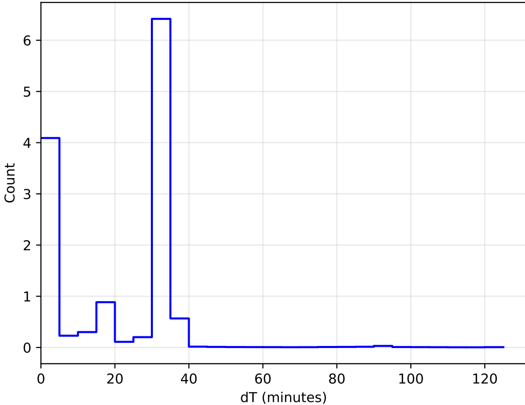
roll_pause_mjdp365_v3.4_10yrs All sky: DeltaT Histogram 1e6
