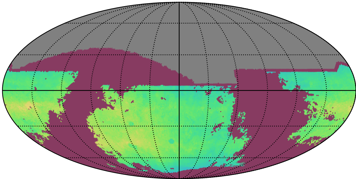
roll_pause_mjdp270_v3.4_10yrs i: NgalScale
