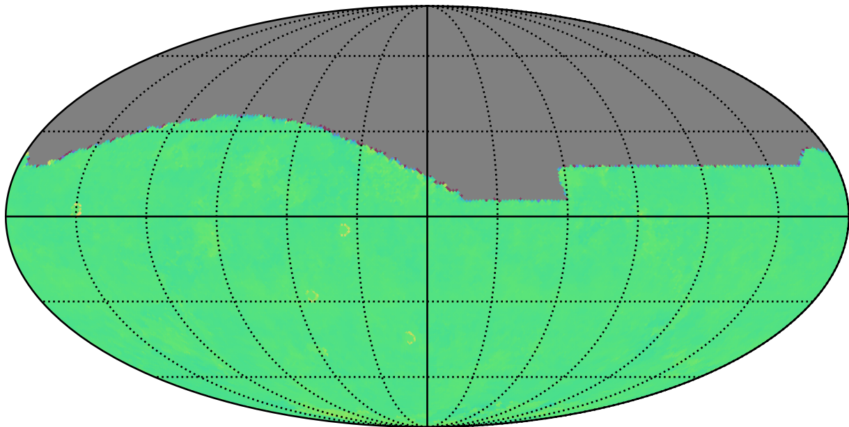
roll_pause_mjdp270_v3.4_10yrs i: Kuiper rotTelPos
