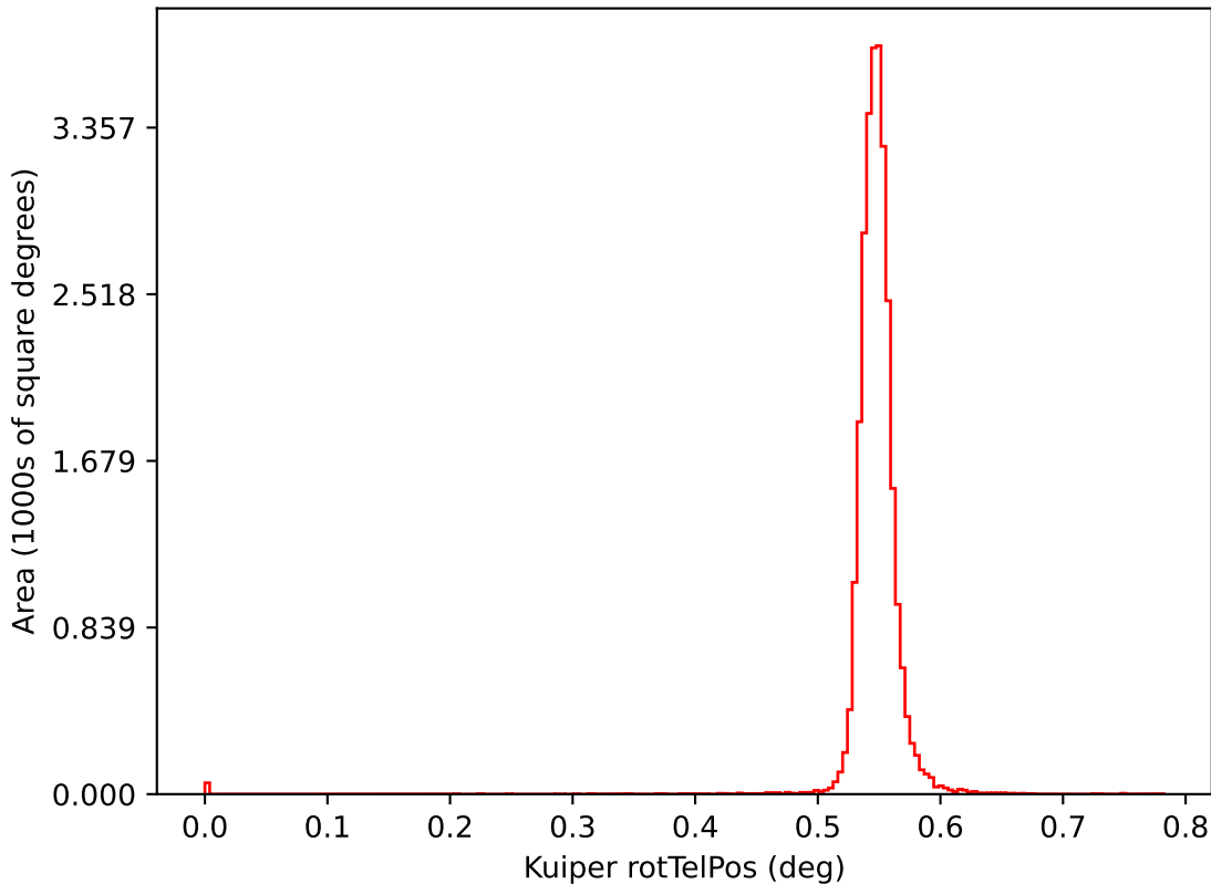
roll_pause_mjdp270_v3.4_10yrs i: Kuiper rotTelPos
