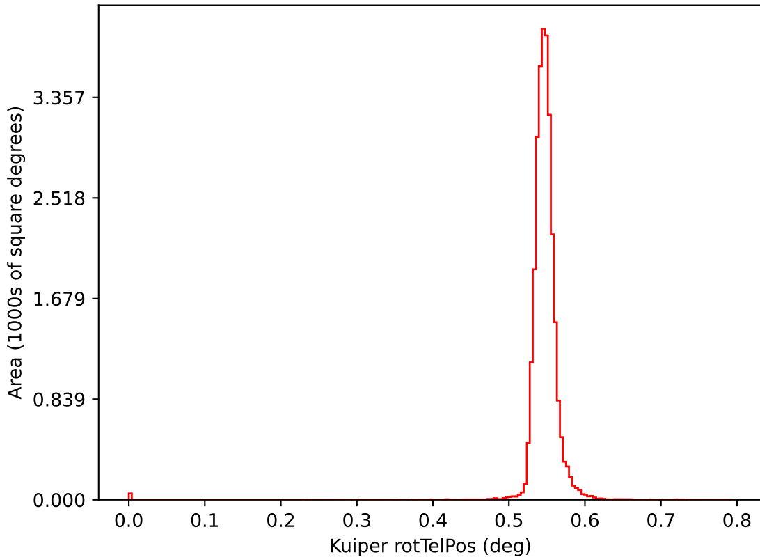
roll_pause_mjdp180_v3.4_10yrs i: Kuiper rotTelPos
